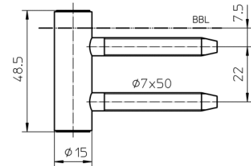
Vorderansicht
