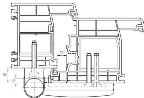
Querschnitt
