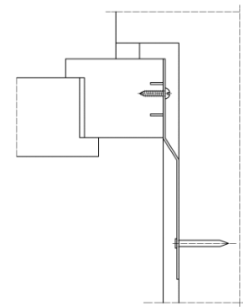
Querschnitt 1
