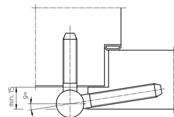
Querschnitt
