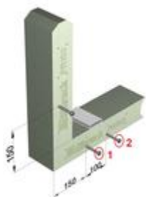
zwei Schrauben verdoppeln die Lastaufnahme je Lasteintragungspunkt
