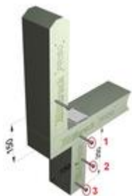
zusätzlicher Stützklötz ab 120mm Ausladung
