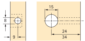
Rastex 15 für 18 mm Fachboden
