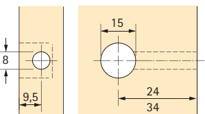
Rastex 15 für 19 mm Fachboden
