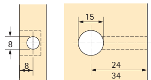
Rastex 15 für 16 mm Fachboden
