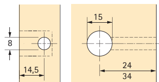
Rastex 15 für 29 mm Fachboden
