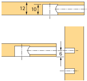
Rastex 15 für 19 mm Fachboden
