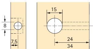
Rastex 15 für 15 mm Fachboden
