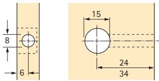
Rastex 15 für 12 mm Fachboden
