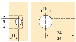
Rastex 15 für 22 mm Fachboden
