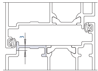
Sperrbügel
