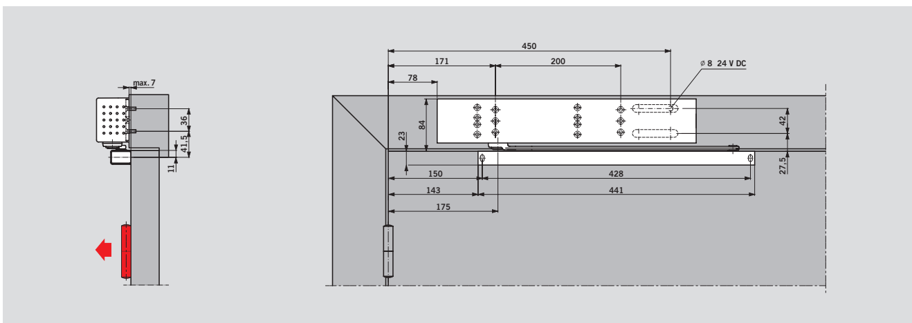
Türschließer TS 99 FL in Kopfmontage (Sturzmontage)
