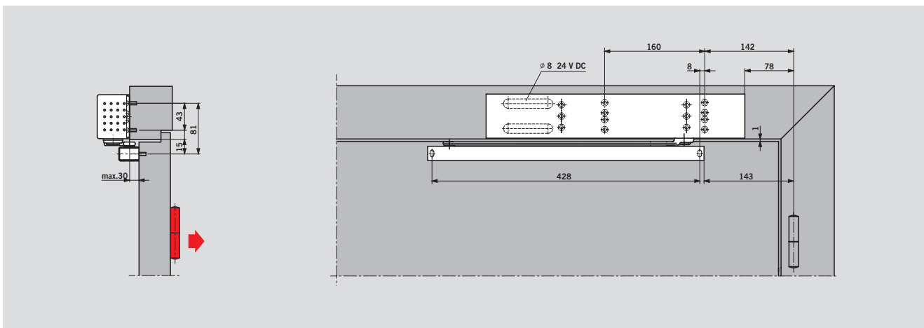
Türschließer TS 99 FL in Kopfmontage auf der Bandgegenseite (Sturzmontage)
