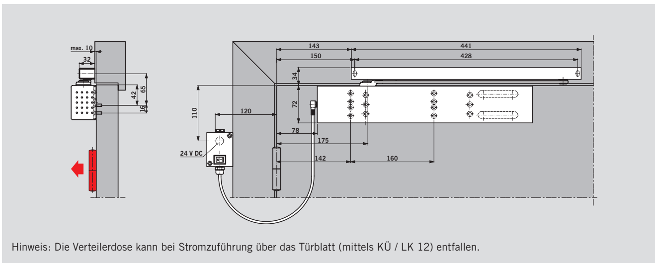
Türschließer TS 99 FL in Normalmontage (Türblattmontage)
