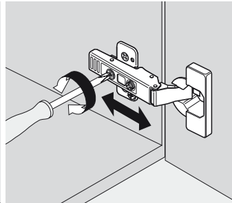
Verstellung Tiefe
