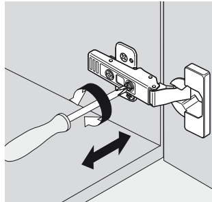
Verstellung Seite
