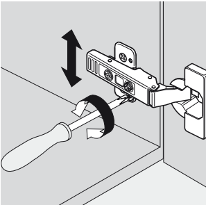
Verstellung Höhe
